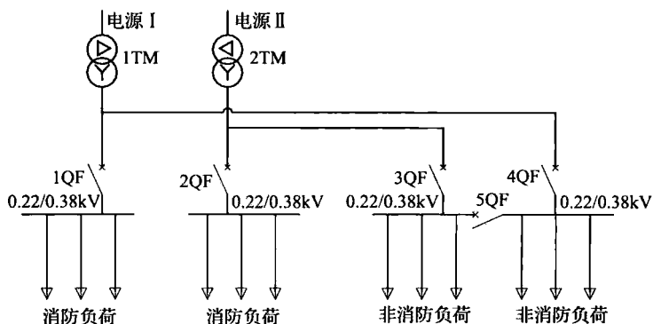
负荷分组设计方案 (二)
