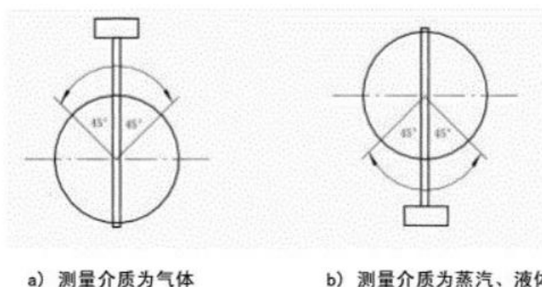
图 7.6.16 均速管流量计插入方位示意
