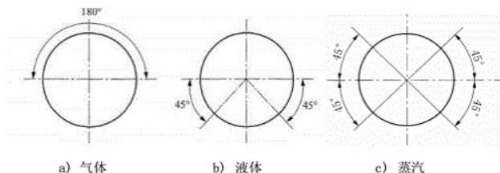
图 7.5.4 压力取源部件的安装方位
