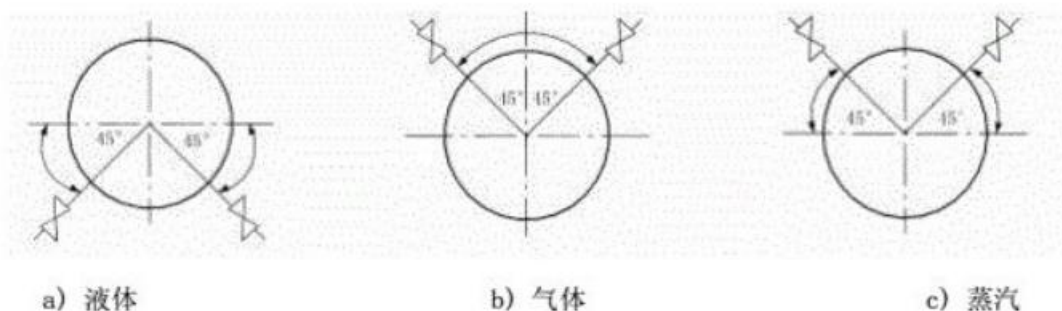
图 7.6.3 节流装置取压孔方位示意
