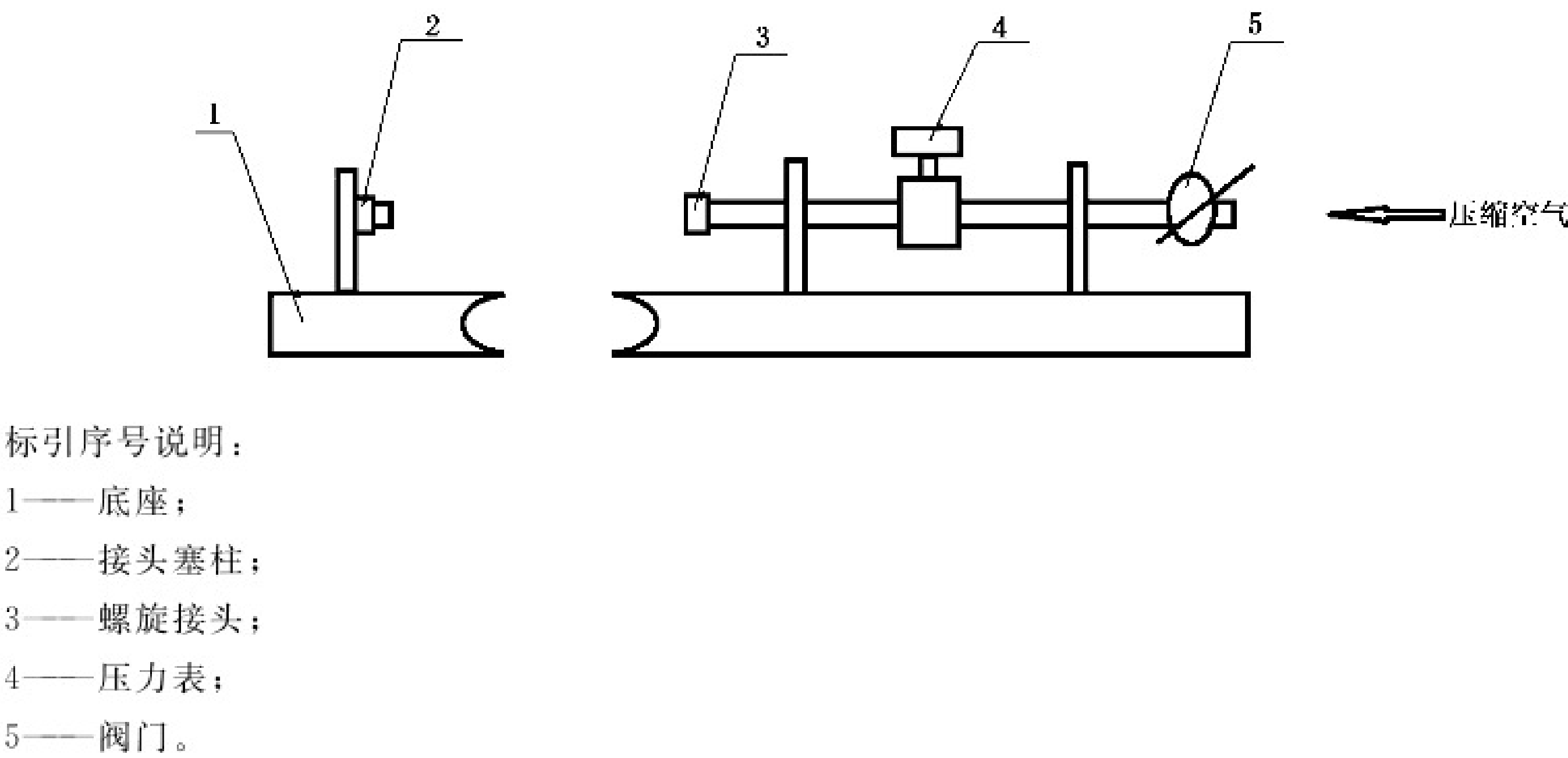
图 D.7 呼吸导管气密性测试装置示意图
