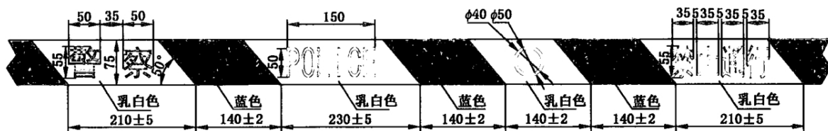
图 1 带体尺寸图
