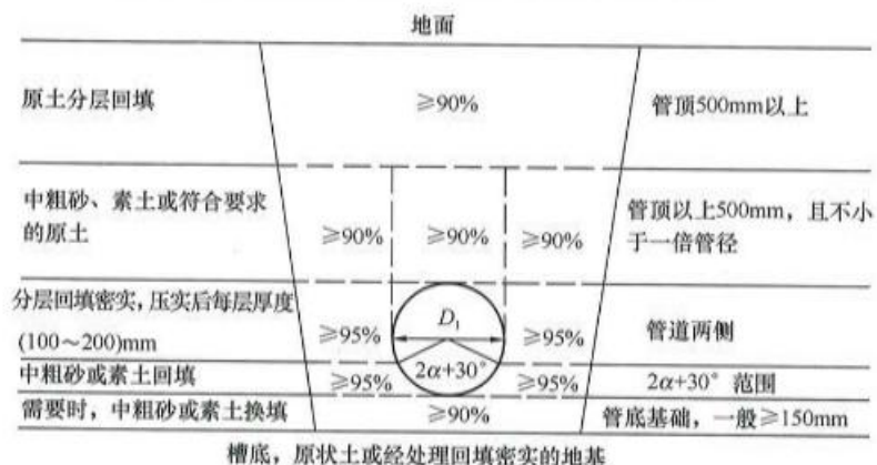
图 2 沟槽回填土压实系数和回填材料示意图
