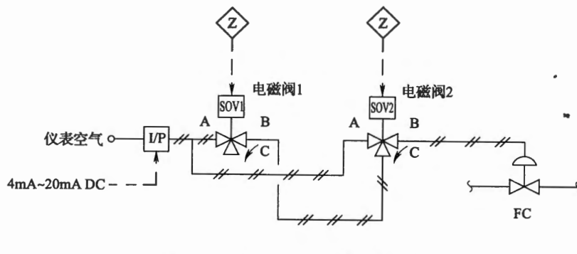
图6 调节阀带冗余电磁阀配置示例
